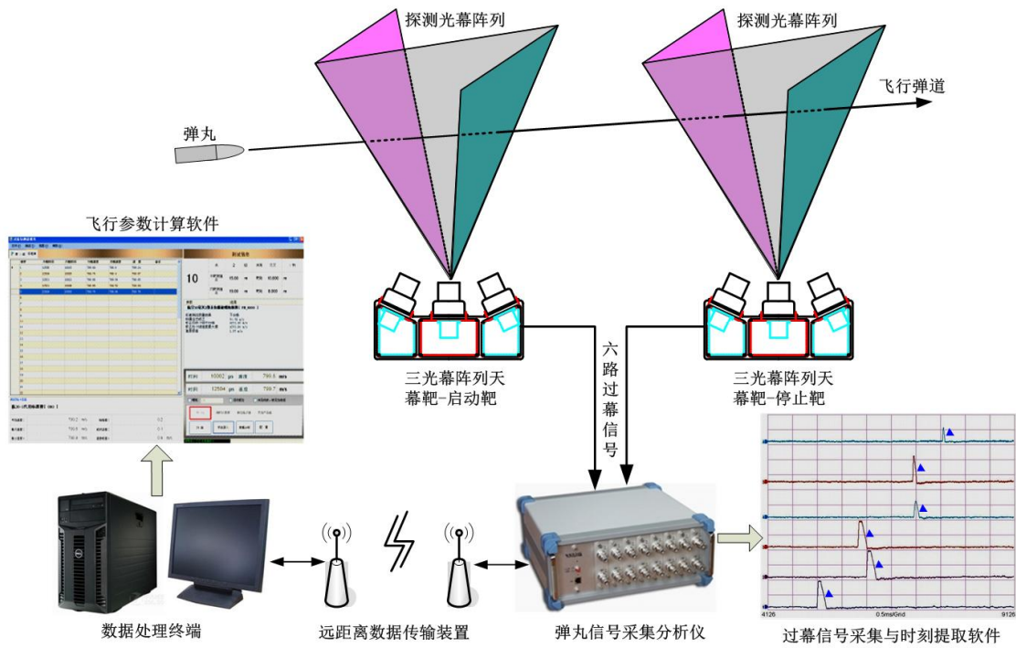
天幕立靶测试系统示意图
